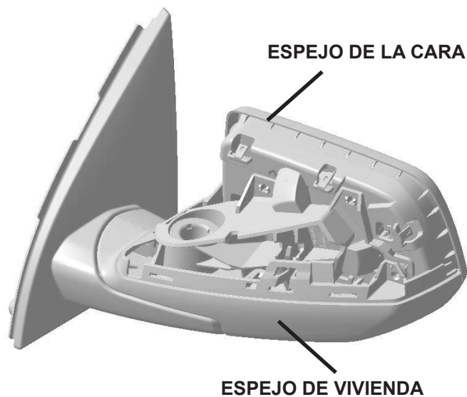
FIGURA 3A – Base del espejo sin la cubierta
