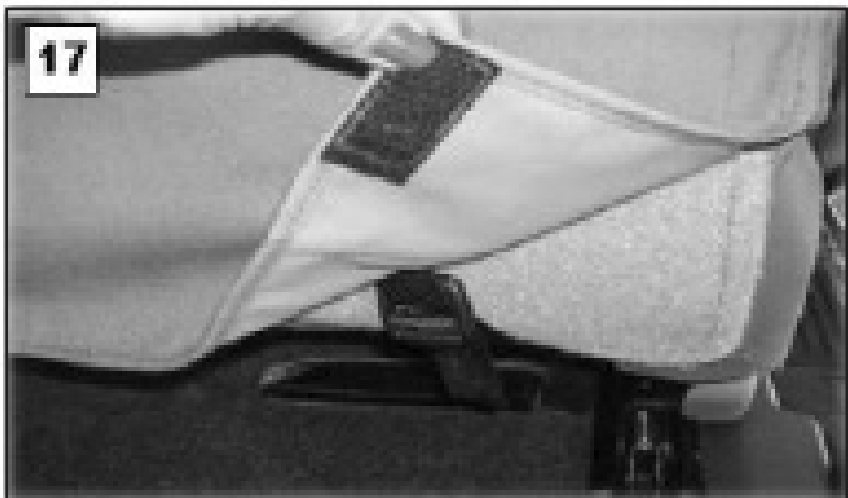
Fixer la bande velcro sur la partie revêtue de moquette du dossier de siège.
