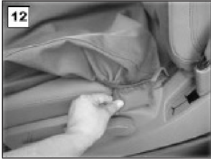
Sujete la almohada al lado del marco del asiento Inserte la almohada detrás de la protección lateral
