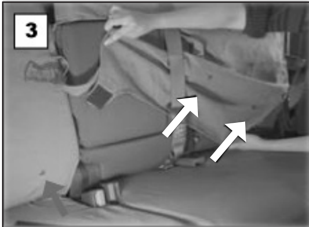
Alinee la abertura y coloque el lazo de tejido
