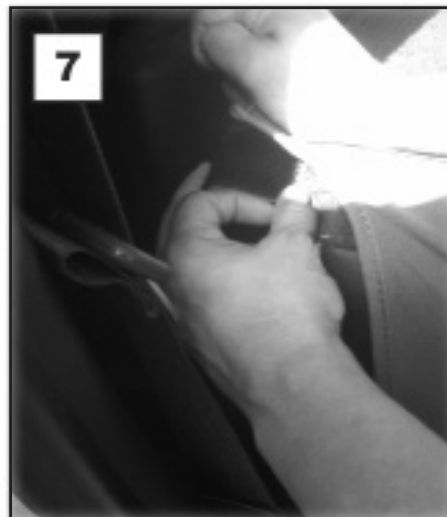
Fixer les bandes velcro à la housse de siège.
